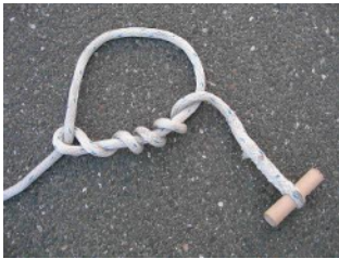
Bild 2: Mastwurf gestochen mit Spierenstich:
